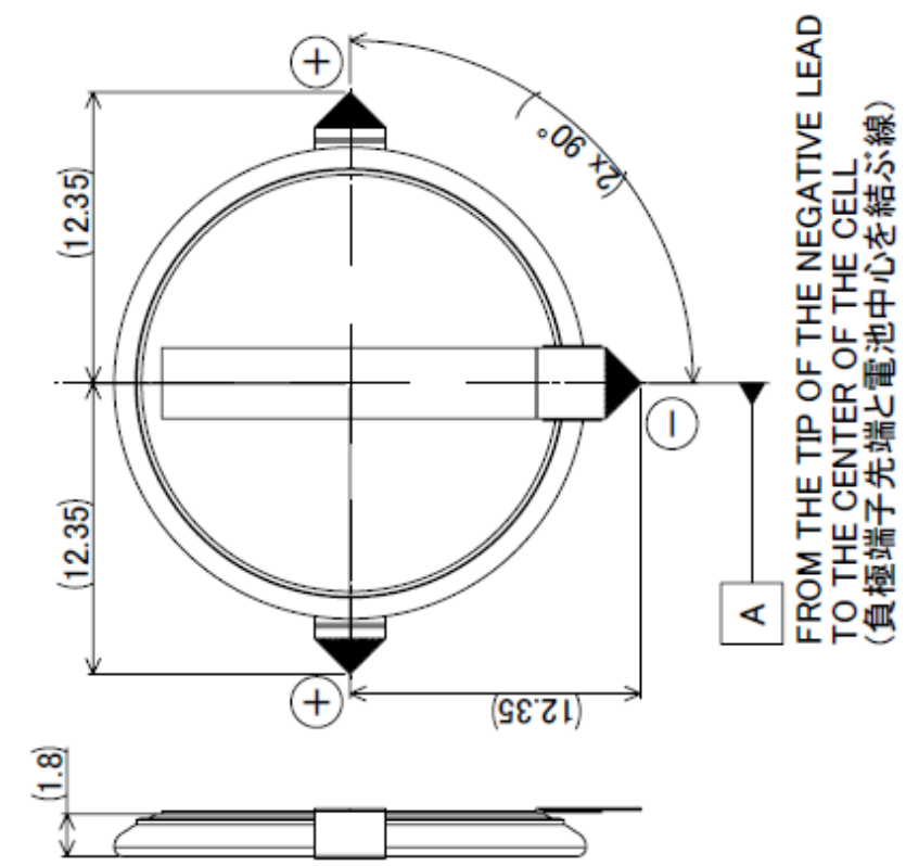
外形図
