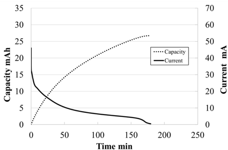
— CV 充電特性(25°C) —
